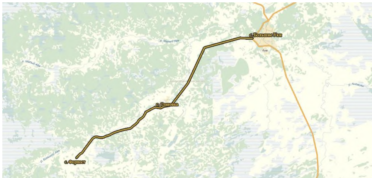
Рисунок №1 Маршрут экскурсии
